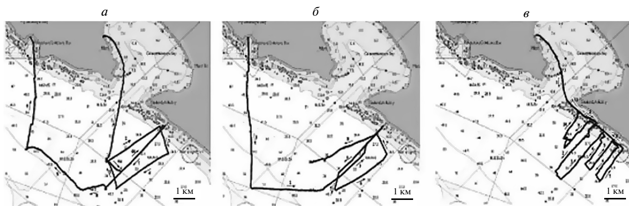
Рис. 2. Схемы галсов, выполненных на Геленджикском шельфе с помощью буксируемого ADCP: а – 1 октября, б – 4 октября, в – 10 октября 2009 г.
