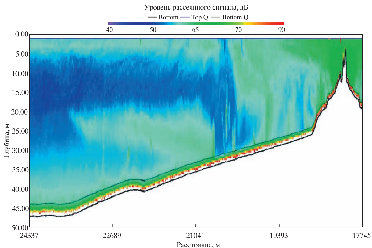
Рис. 4. Интенсивности рассеянного акустического сигнала по данным измерений 1 октября 2009 г. вблизи сбросового устройства: вверху – цветовая шкала интенсивности рассеянного сигнала в децибелах; внизу – отражения от рельефа дна.
