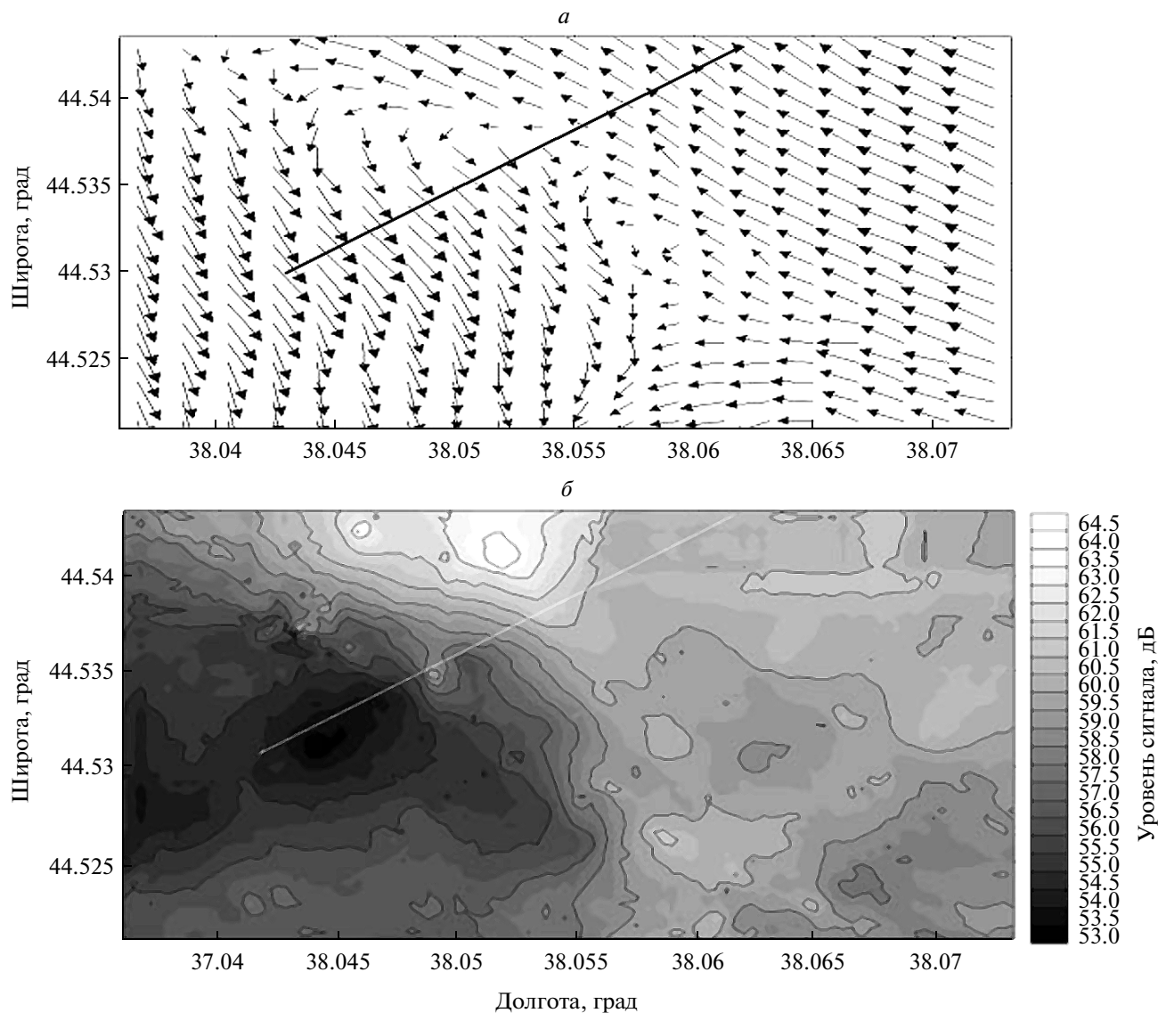
Рис. 6. а – Карта векторов баротропных течений 10 октября 2009 г.; б – карта уровня обратного рассеяния акустического сигнала в дБ. Положение трубопровода глубоководного стока показано белой линией.
