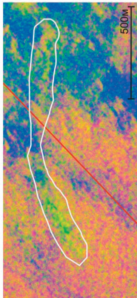
Рис. 8. Фрагмент исходного космического изображения, полученного со спутника IKONOS, для района расположения сбросового коллектора: а и б – результат декорреляционного растяжения данного фрагмента изображения; в и г – увеличенные фрагменты изображения б .
